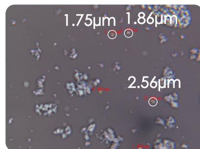
伊利石干法研磨后电镜图
