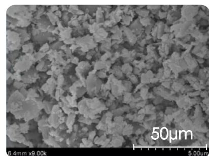
铈酸锂研磨后电镜图
